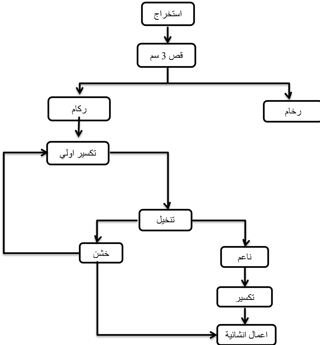
رسم توضيحي 3 مخطط سير عمليات معالجة خام الرخام
